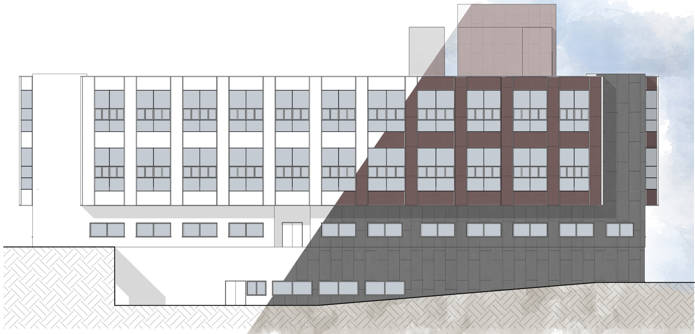
PP_ARC_1:200_Prospetto Sud_SDP
