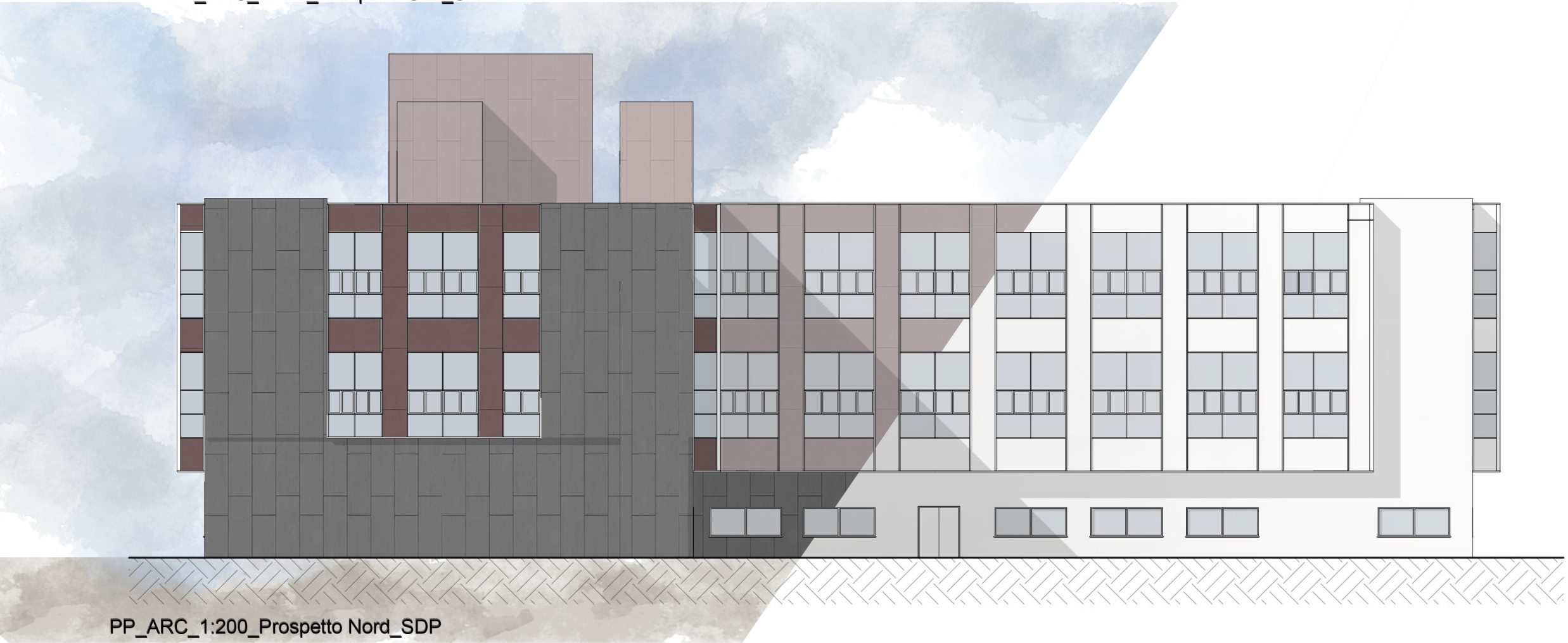
PP_ARC_1:200_Prospetto Nord_SDP
